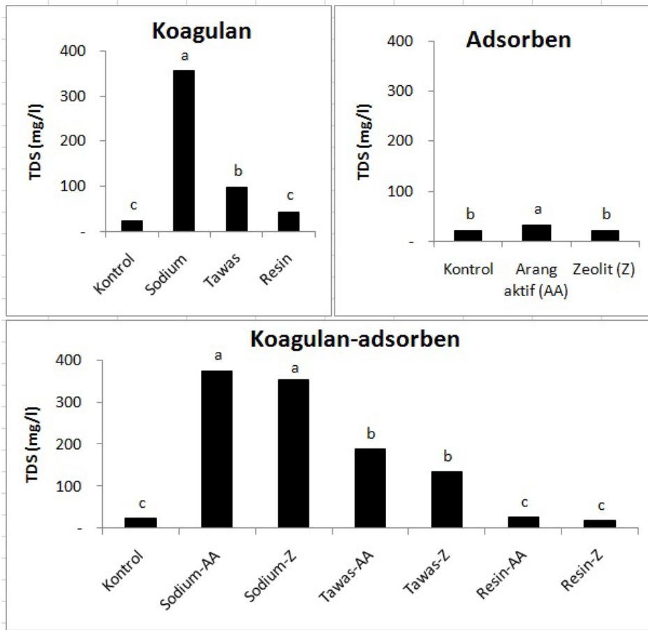
Gambar 4. Pengaruh Koagulan, Adsorben, dan Kombinasi Koagulan-Adsorben Terhadap TDS Limbah Cair Electroplating
